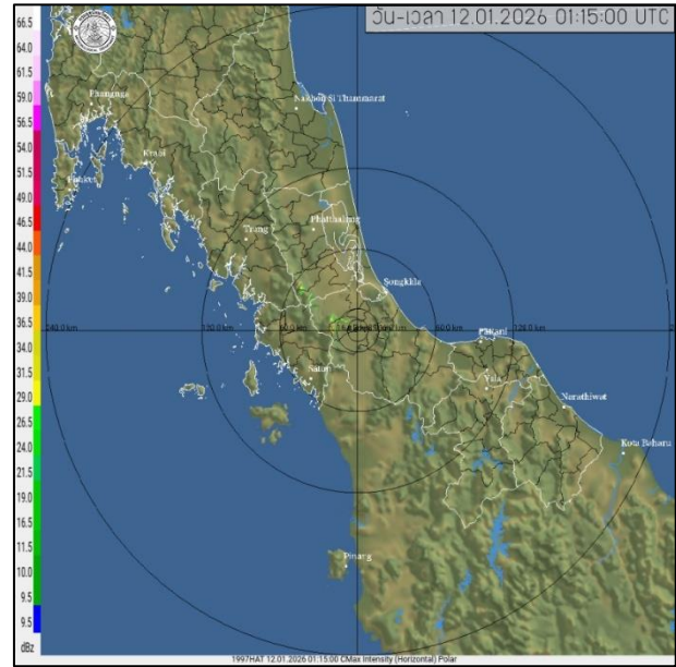
สถานีหาดใหญ่ เวลา ๐๘.๑๕ น.
