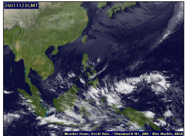
ภาพถ่ายดาวเทียม วันที่ ๑๒ ม.ค. ๒๕๖๙ เวลา ๐๖.๐๐ น.
